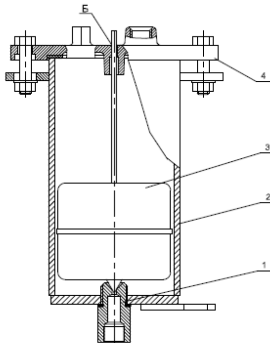
1 - Штуцер. 2 - Корпус. 3 - Поплавок. 4 - Крышка.
