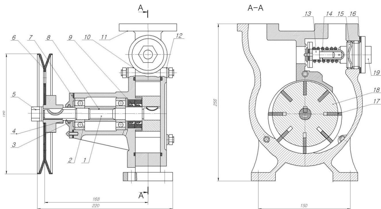
1 - Вал. 2 - Подшипник. 3 - Кольцо. 4 - Втулка. 5 - Гайка. 6 - Шкив. 7 - Крышка подшипника. 8 - Втулка распорная. 9 - Манжета. 10 - Крышка. 11 - Корпус. 12 - Крышка задняя. 13 - Клапан. 14 - Пружина. 15 - Винт регулировочный. 16 - Прокладка. 17 - Лопатка. 18 - Ротор. 19 - Пробка.
