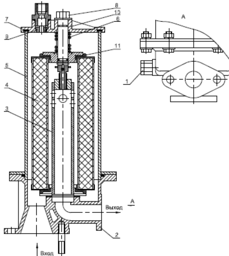
1 - Пробка. 2 - Корпус. 3 - Труба. 4 – Фильтрующий элемент. 5 - Корпус. 6 - Пружина. 7 - Прокладка. 8 - Винт. 9 - Втулка. 10 - Крышка. 11 – Кольцо.
